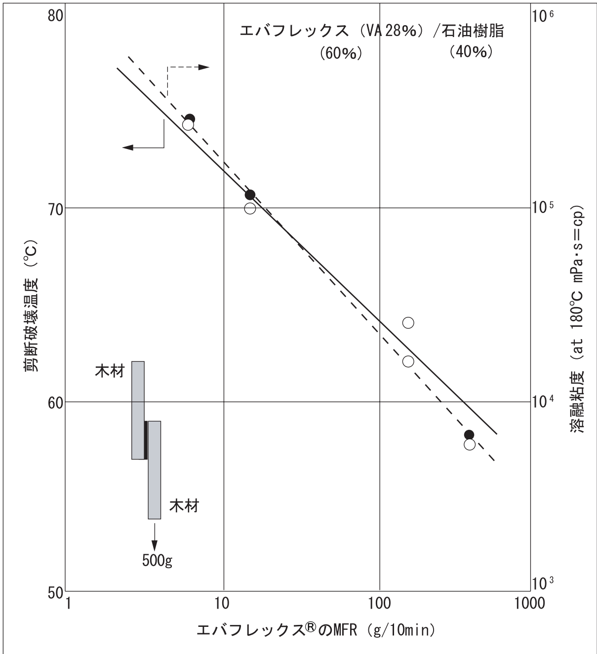
図3 ホットメルト配合物の耐熱接着性に及ぼすエバフレックス®のMFRの影響
