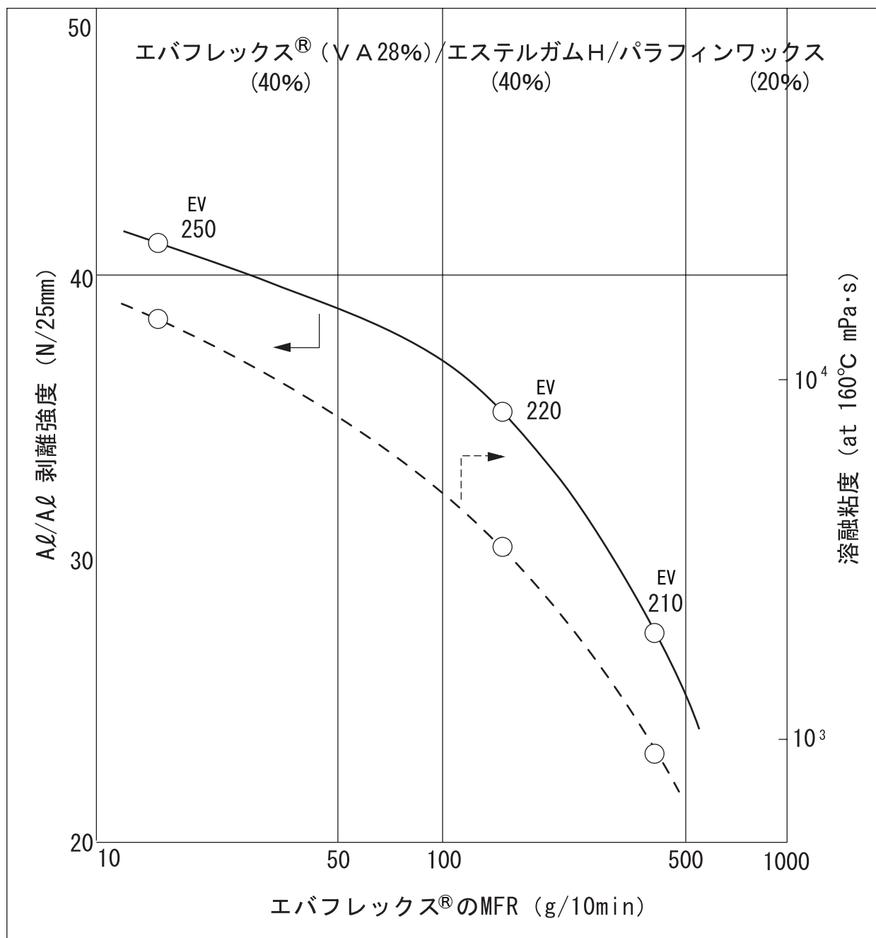
図2 ホットメルト配合物の接着性に及ぼすエバフレックス®のMFRの影響
