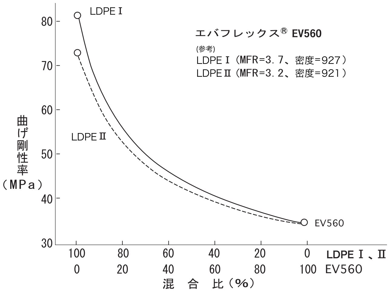
図2 低密度ポリエチレン/エバフレックス®ブレンド系の曲げ剛性率 (測定法 JIS K7106)
