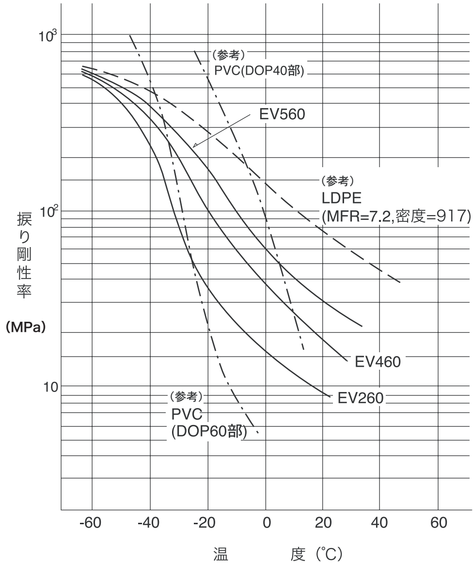
図一 振り剛性率—温度曲線 (測定法 ASTM D-1043)
